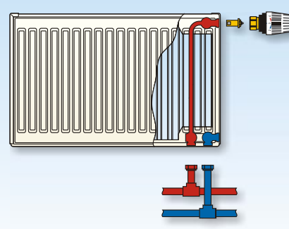
Pripojenie vpravo
